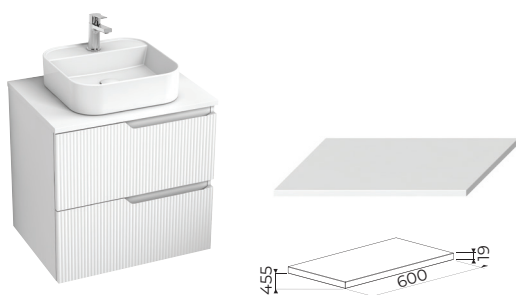
Vrchní deska pro skříňky H40J441, 60 cm pod umyvadlovou mísu, (bez otvoru pro sifon) H46J441220xxx1
