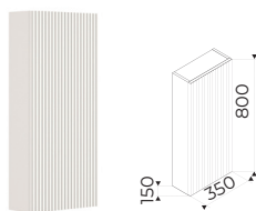
Střední mělká skříňka, 1 dveře levé/pravé, 2 skleněné police H43J444130xxx1
