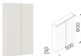
Střední mělká skříňka, 2 dveře levé/pravé, 2 skleněné police H43J441200xxx1
