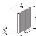
Skříňka pod umývatko 45 cm, 1 dveře H40J445102xxx1
